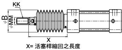
軸附防塵套氣缸(FCL-H)
