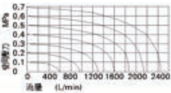
型號: W4V310-10
