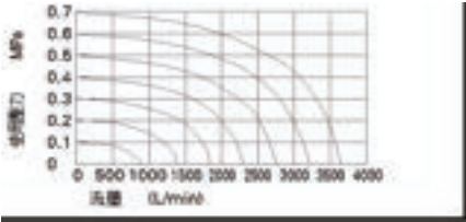
型號：W4V410-15
