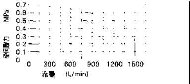
型號: W4V210-08
