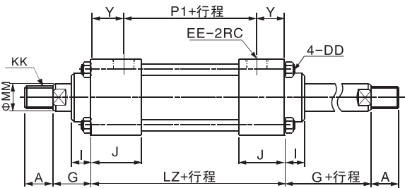
軸附防塵套油缸(HC.A-H)
