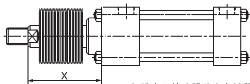
軸附防塵套油缸(HC.A-H)
