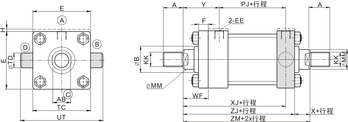
MT2(TB) 雙軸缸后砲耳型
