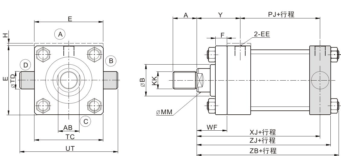
MT2(TB) 複動缸后砲耳型
