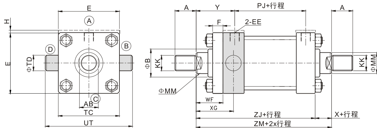
MT1(TA) 雙軸缸前砲耳型
