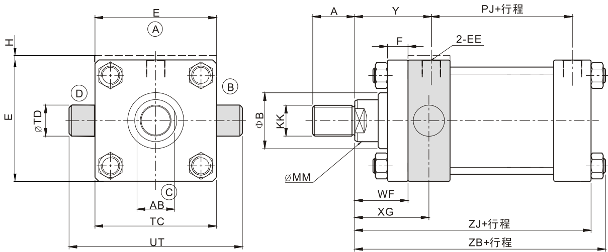
MT1(TA) 複動缸前砲耳型
